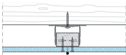
Joint > 1mm (éliminer l'excédent de colle)
